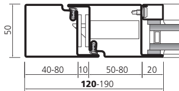
Nicht isolierte Tür Porte sans isolation thermique Door without thermal break
