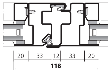
Nicht isoliertes Fenster Fenêtre sans isolation thermique Window without thermal break
