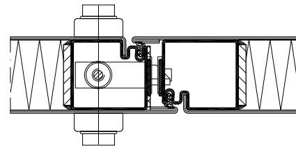
Verblechte Rohrrahmen-tür Porte en tôle d'acier Sheet metal door
