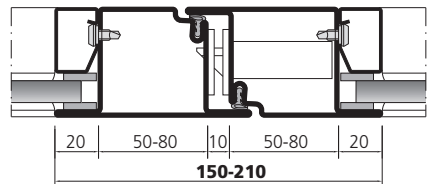
Rauchschutztür Porte pare-flamme Smoke protection door
