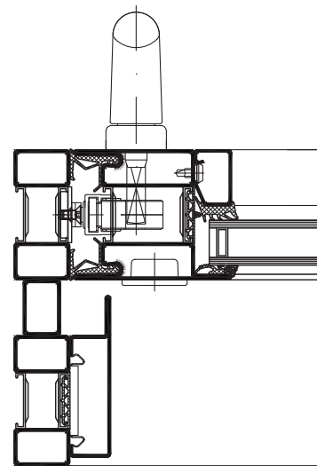
Hebeschiebetür Porte coulissante à levier Lift-up sliding door
